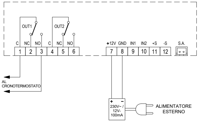
Fig. 8: Esempio di collegamento ad un cronotermostato.
