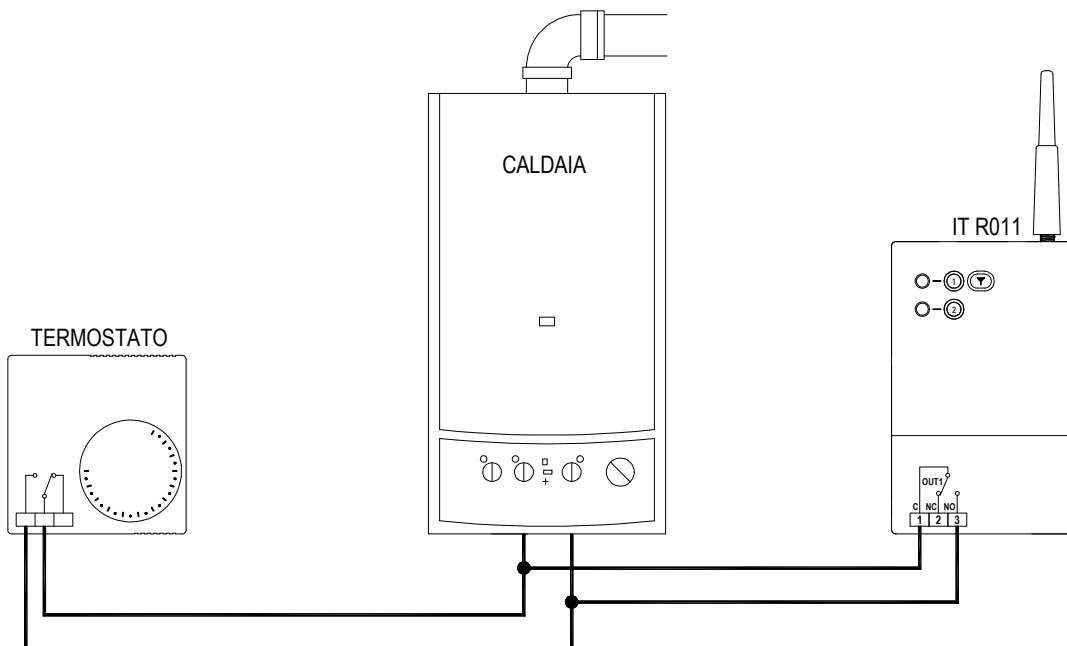
Fig. 10: Esempio di un collegamento in parallelo dell'interfaccia telefonica con un termostato.
